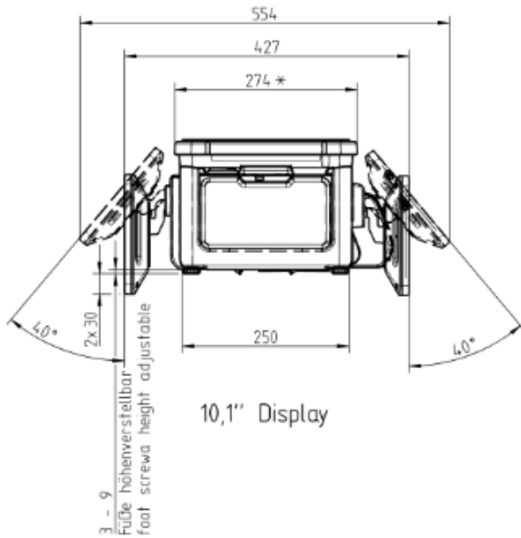
Q1_expert_100_side_view_10,1_display_01
