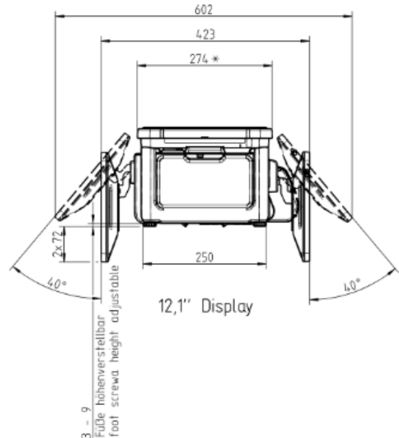
Q1_expert_100_side_view_12,1_display_01
